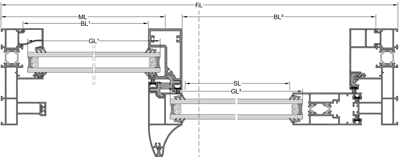
A-A KESİTİ
