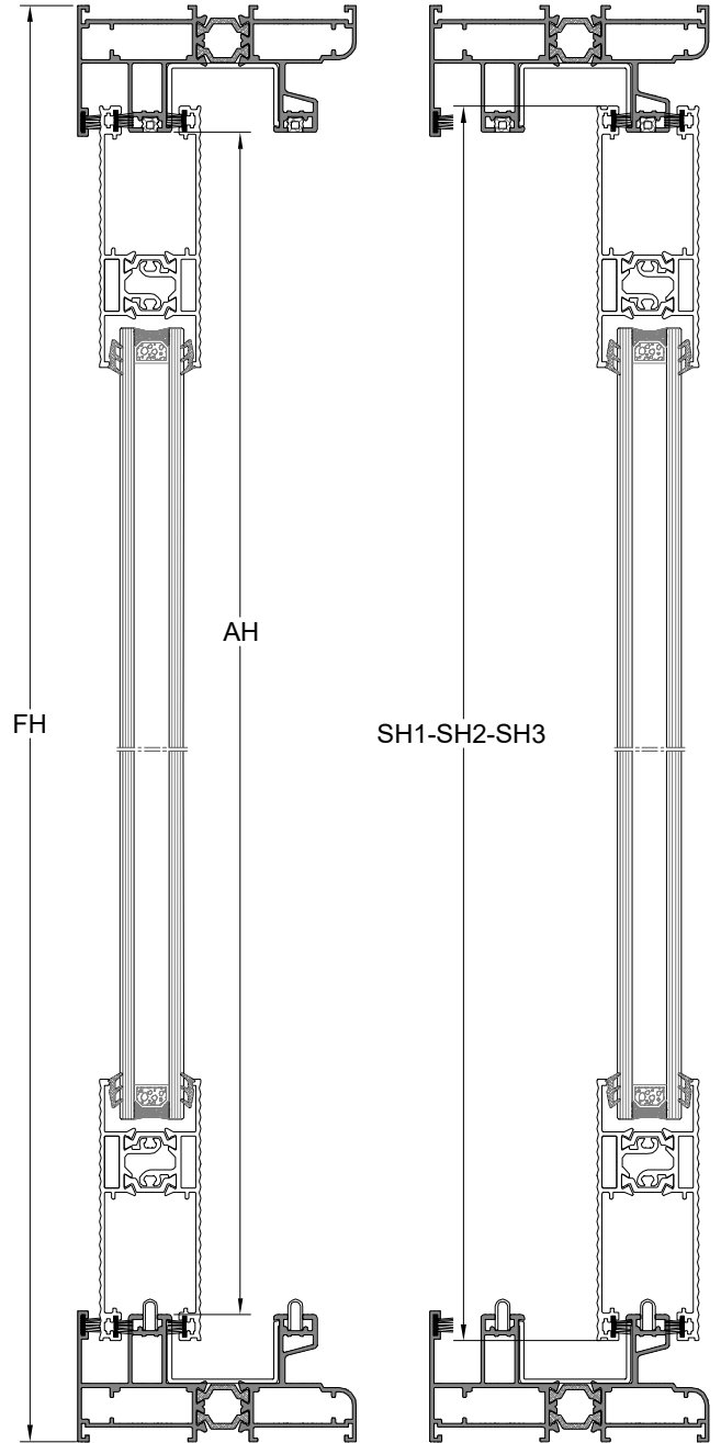
B-B KESİTİ
